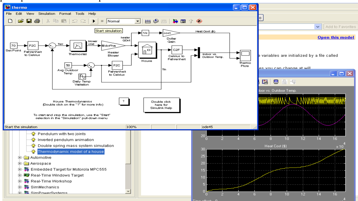
Рис.2. Термодинамическая модель дома
